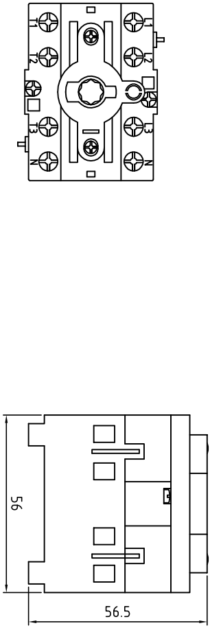
Anschlußbild
